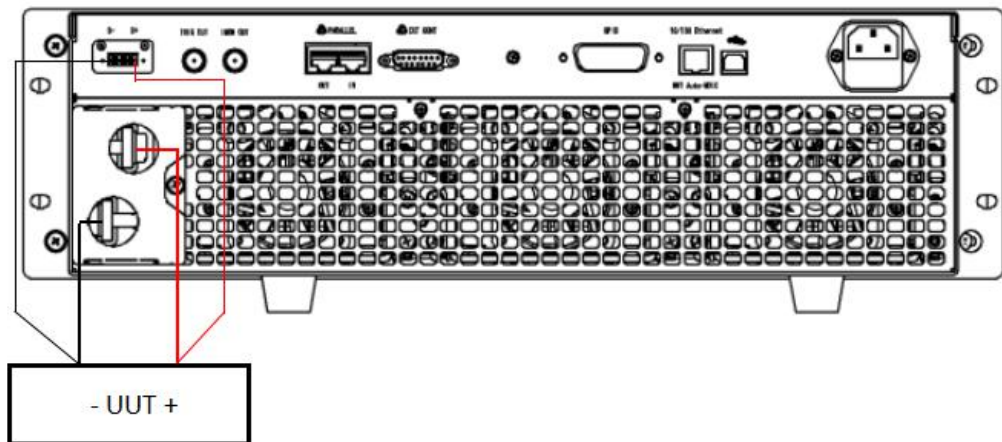
图 3-2 遥测操作连接
