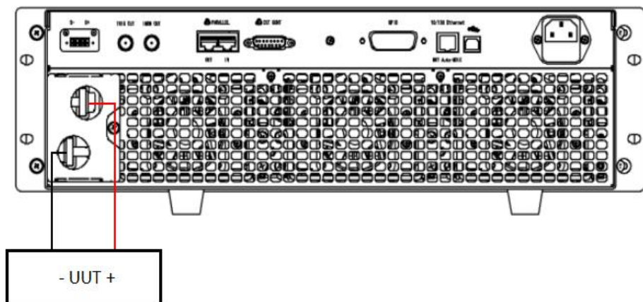
图 3-1 负载接线示意图
