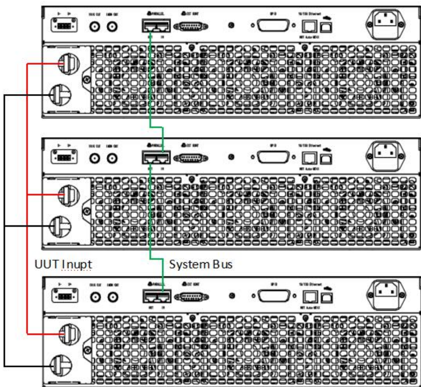
图 3-3 并联式连接
