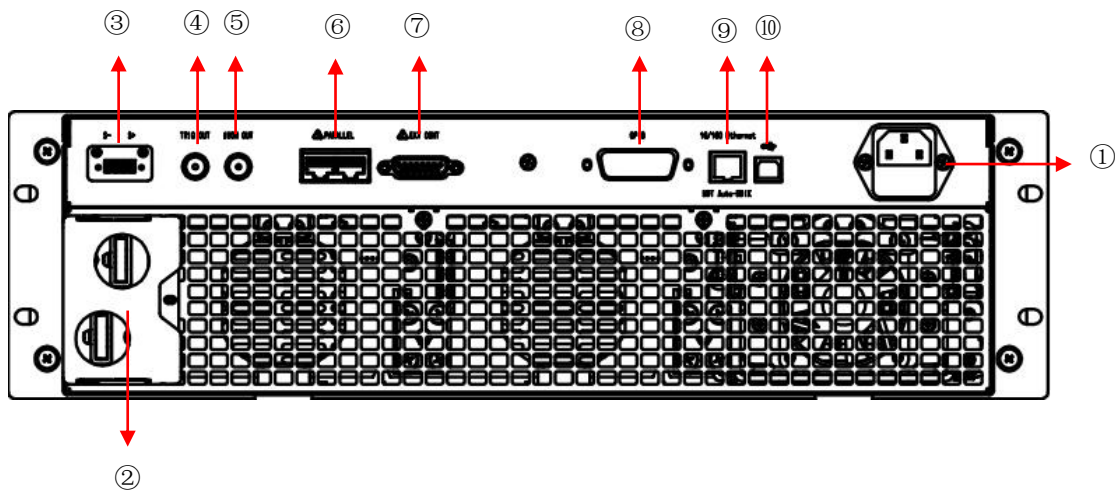
图 2-2 电子负载的后面板
