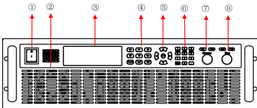
图 2-1 电子负载的前面板
