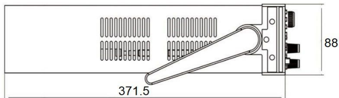
图 2.2.2 DH1765 侧视图（单位：mm）
