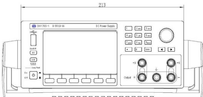
图 2.2.1 DH1765 正视图（单位：mm）
