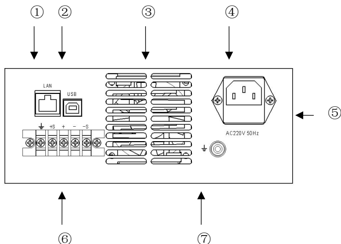
图 5.2.1 DH1766 后面板示意图
