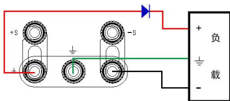
图 6.5.4 串联二极管示意图
