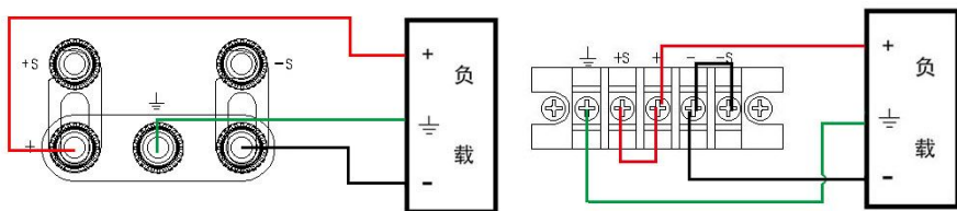
图 5.1.2 负载接线方式示意图
